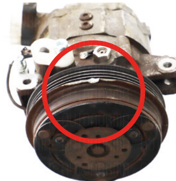
Poškození řemenice kompresoru
